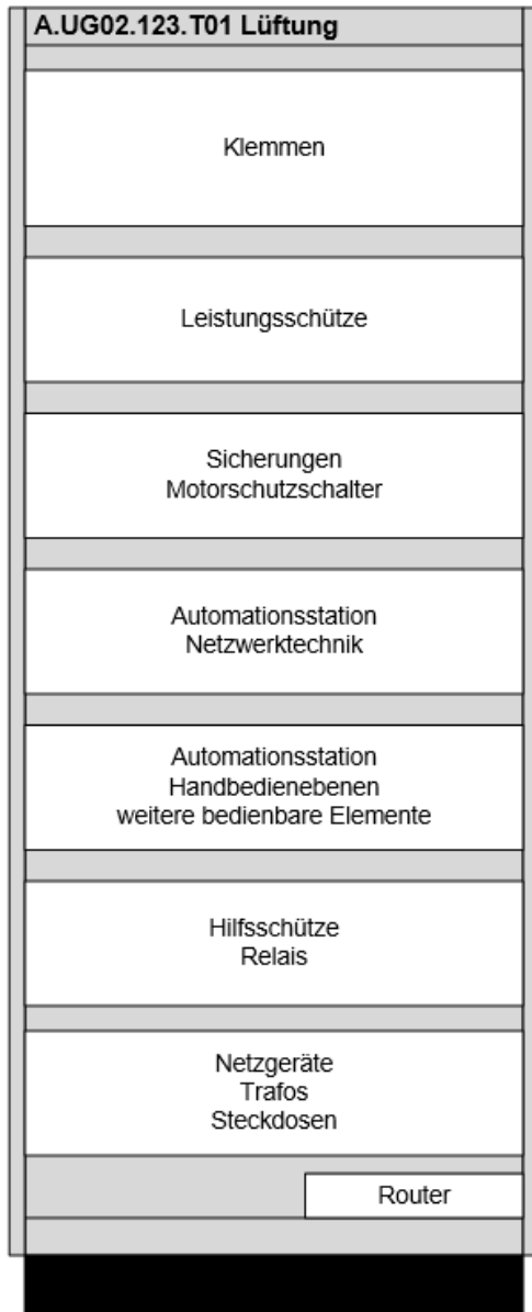
Abbildung 2: Schaltschranklayout innen (Klemmen oben)
